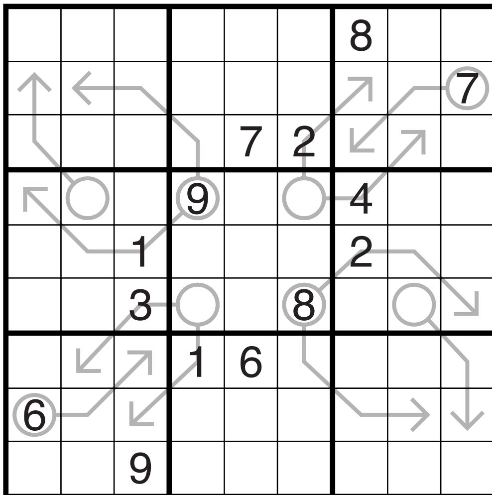
Arrow Entanglement
